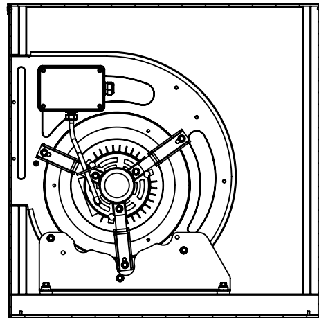
SEZIONE A-A
