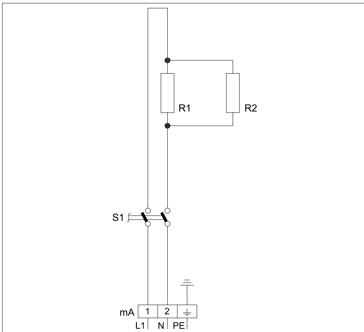
Abb. 18 Stromlaufplan
