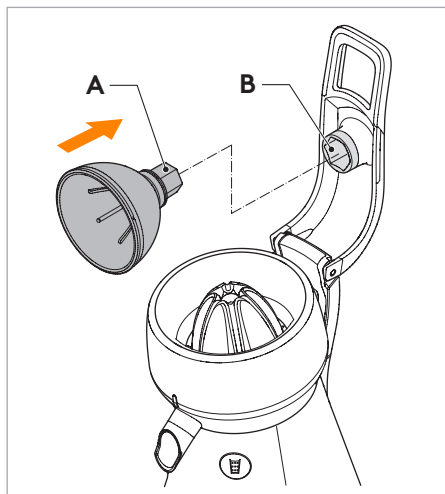
15. Setzen Sie die Pressschale (A) auf den Hebel (B).
