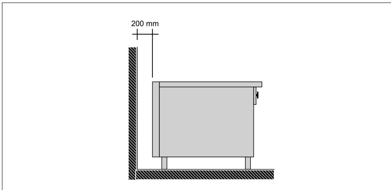
Abb. 10 Minimalabstand von entzündlichen Wänden
