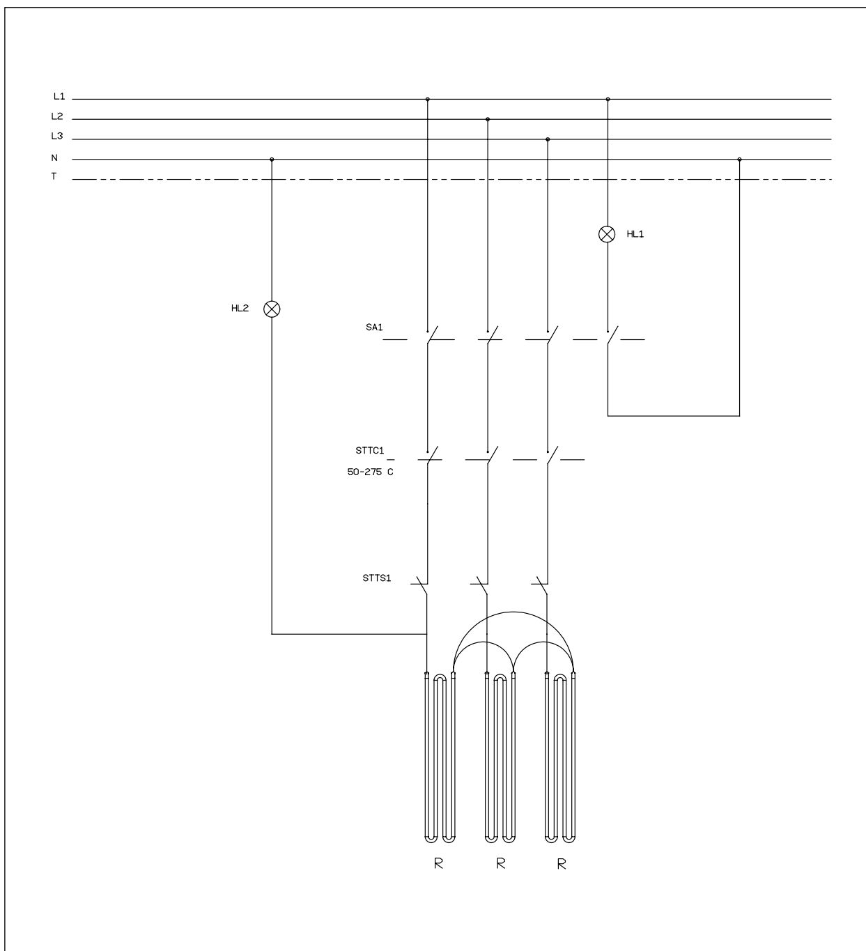
Abb. 13 Stromlaufplan
