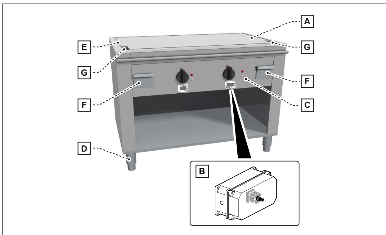
Abb. 3 Hauptteile des Geräts
