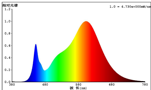
光谱分布
